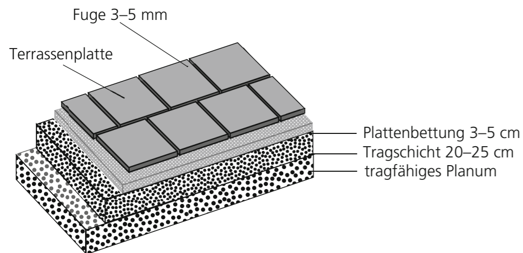
Schematischer Aufbau eines Terrassenplattenbelags (lose Verlegung)
