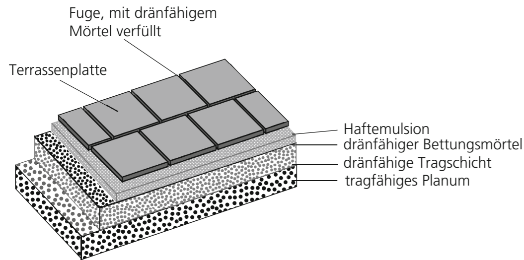
Schematischer Aufbau eines Terrassenbelags auf gebundener Tragschicht (feste Verlegung)
