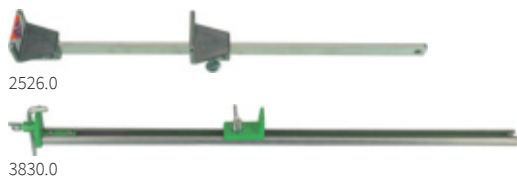
Lattenstichmaß aus Alu mit Meßskala und Schraube
