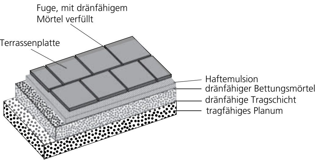
Schematischer Aufbau eines Terrassenbelags auf gebundener Tragschicht (feste Verlegung)
