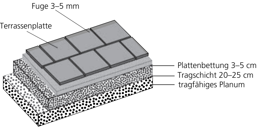
Schematischer Aufbau eines Terrassenplattenbelags (lose Verlegung)
