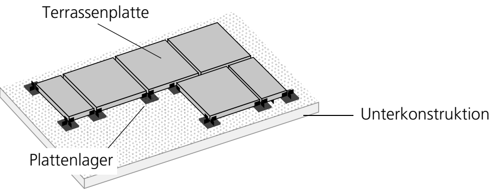
Schematischer Aufbau eines Terrassenbelags auf Plattenlager
