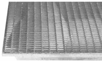
Gitterroste begehbar Maschenweite 30/10 Punktlast 150kg/m 2
